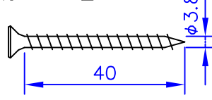
取付ネジ×2
